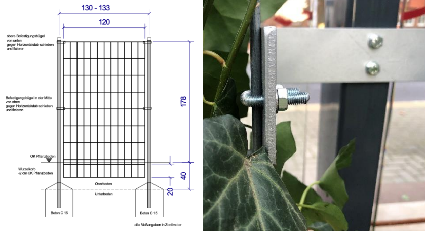
Abbildung 4 Systemskizze für den Einbau und Unterkonstruktion der laufenden Hecke, individuelle Halterungen bei der Schatteninsel
